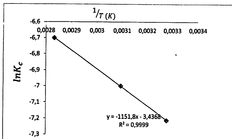
Fig. 11. Plot of \ln K_c vs. 1/T \text{ (K}^{-1}\text{)} .
